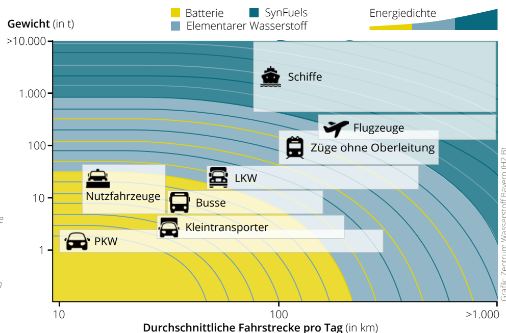
Abbildung 1: Die verschiedenen Antriebstechnologien schließen sich nicht gegenseitig aus. Je nach Gewicht und Fahrstrecke kommen die Vorteile unterschiedlicher Technologien zum Tragen. Grafik in Anlehnung an Hydrogen Council 2017 [8].
