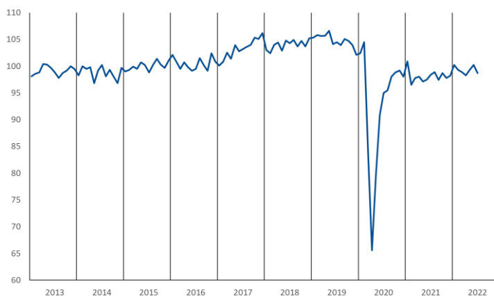
Industrieproduktion, saisonbereinigt, 2010 = 100
